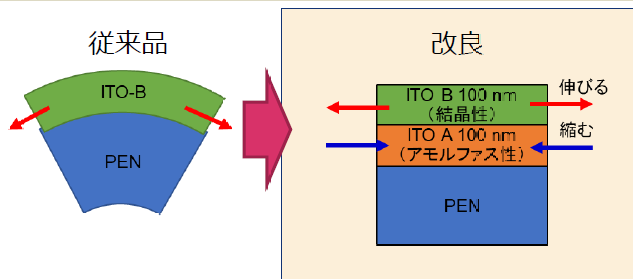
図5 独自の成膜技術
