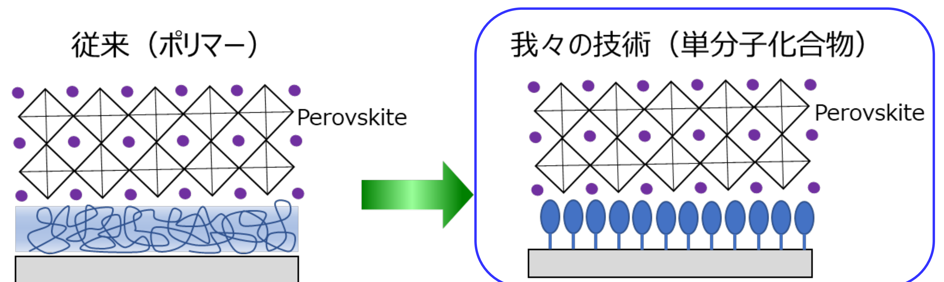
図7 独自の単分子ホール回収層のイメージ図
