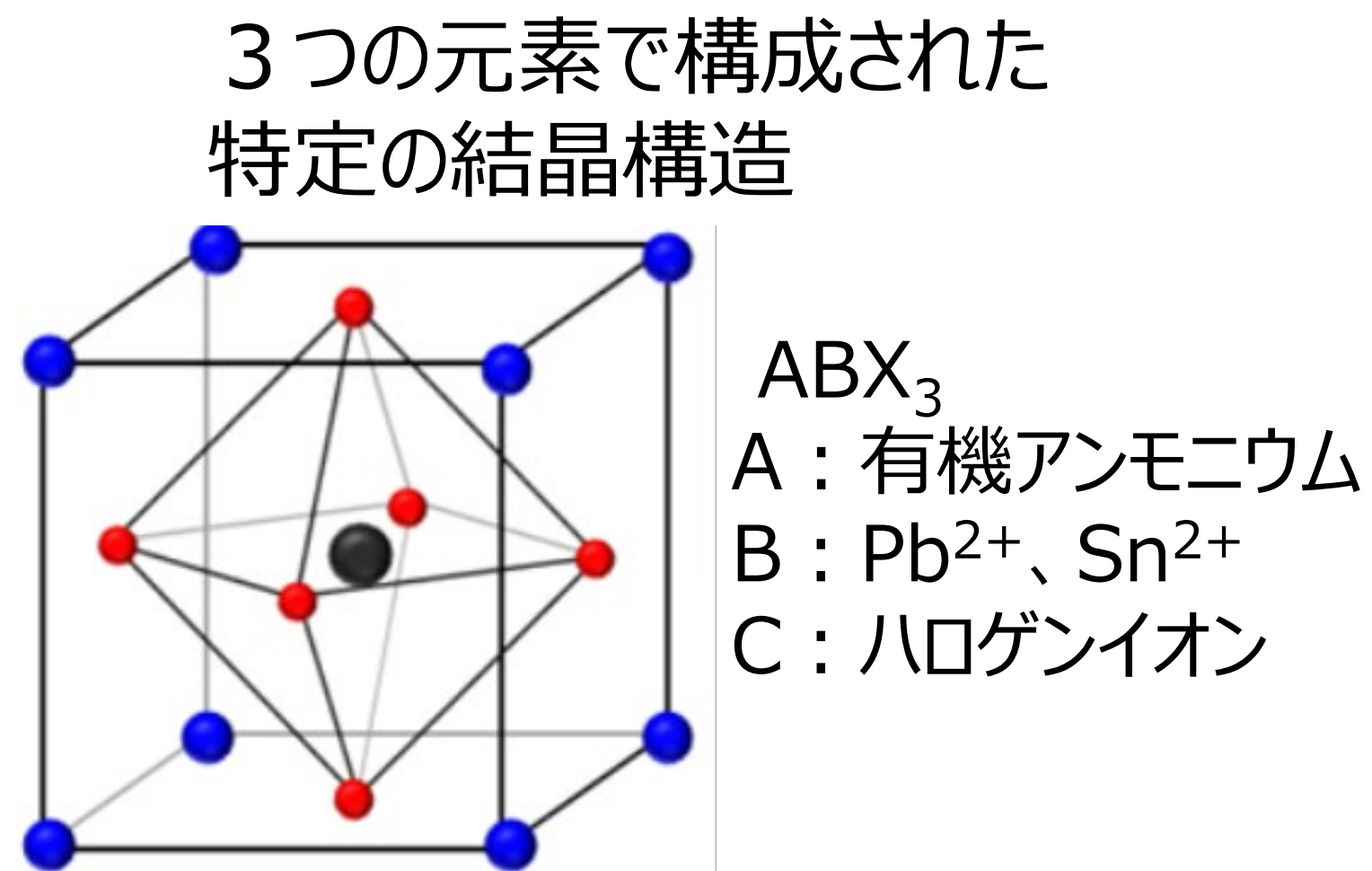
図1 ペロブスカイト結晶の構造
