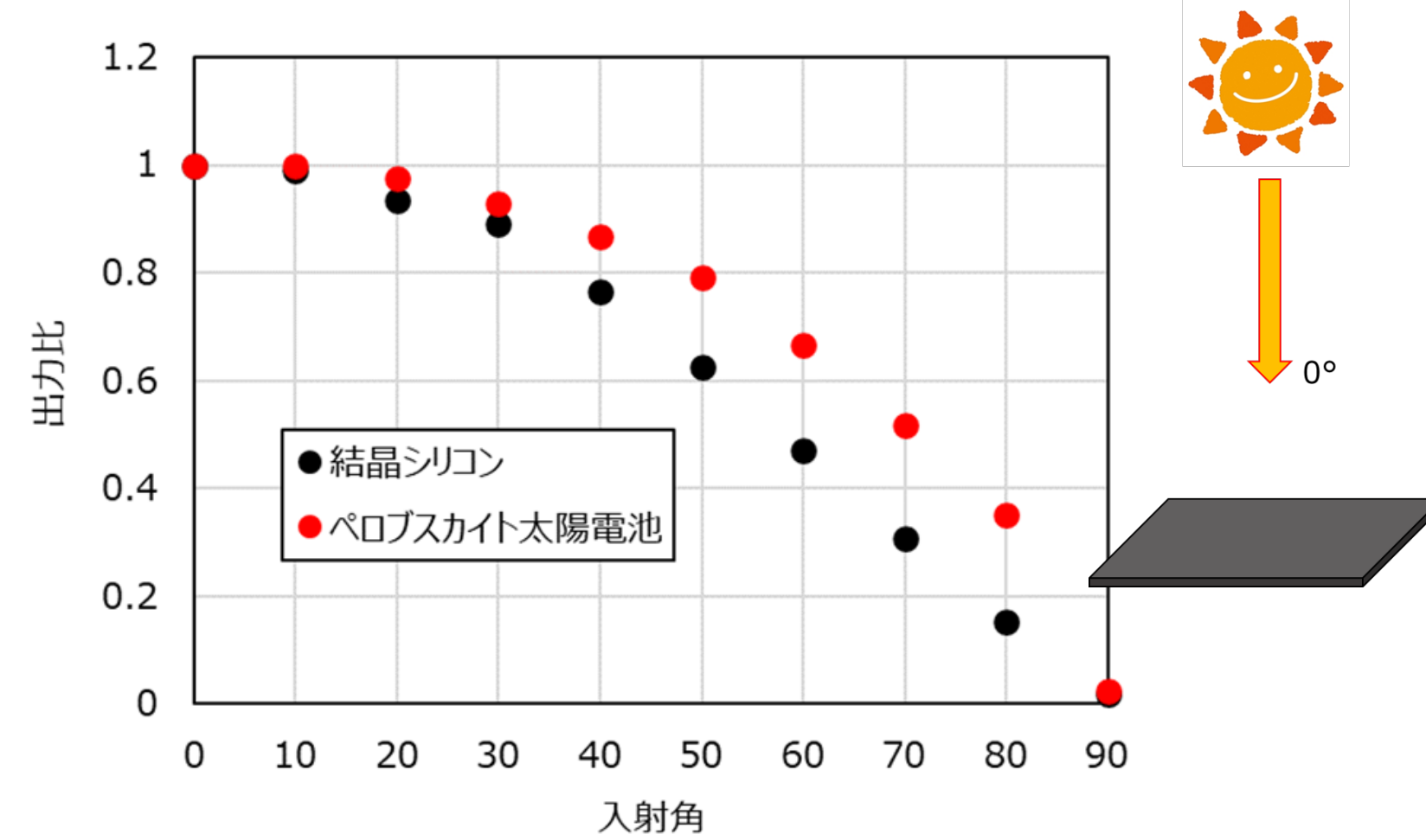
図3 角度依存特性
