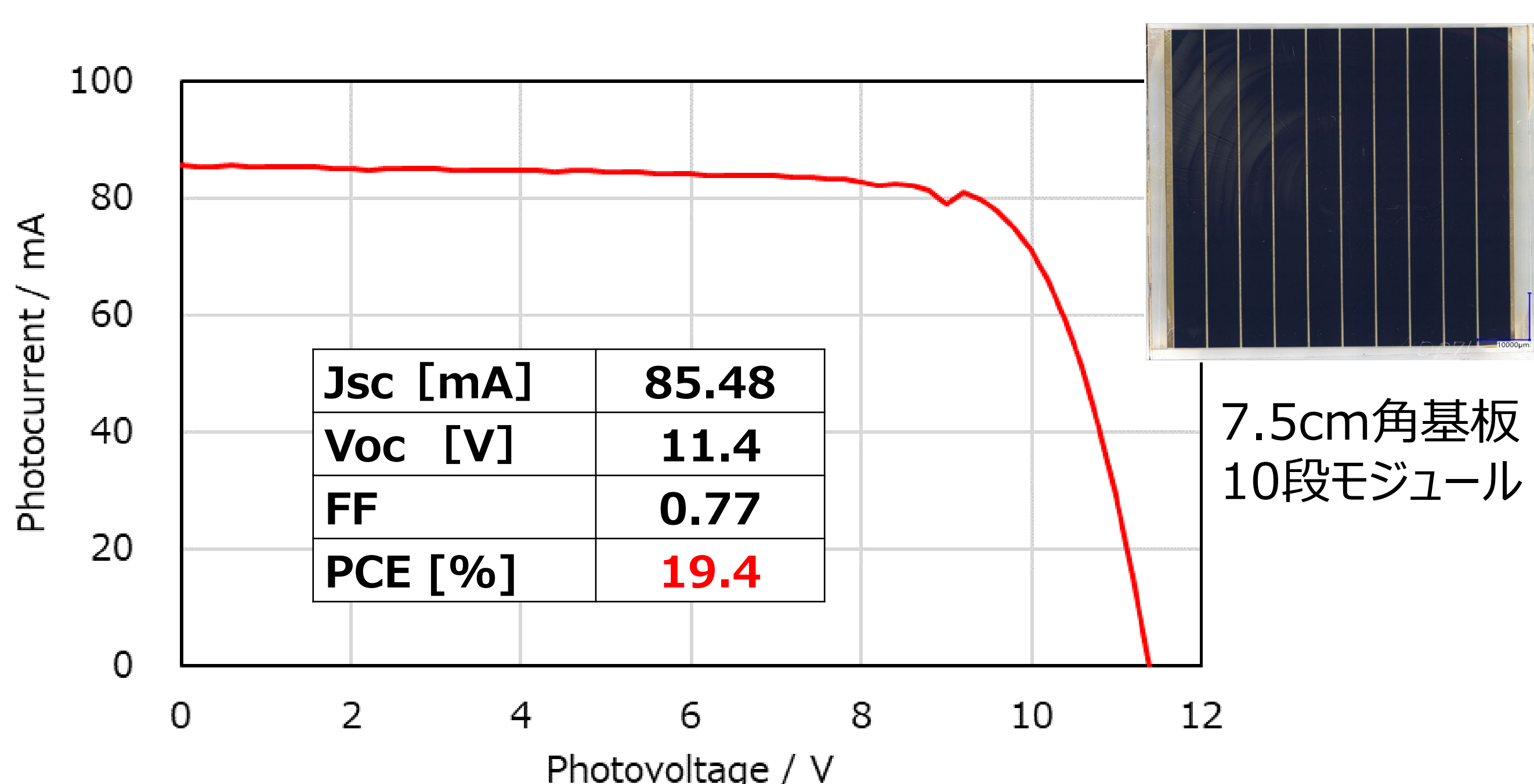
図8 フィルム型ペロブスカイト太陽電池モジュールの特性(1SUN)
