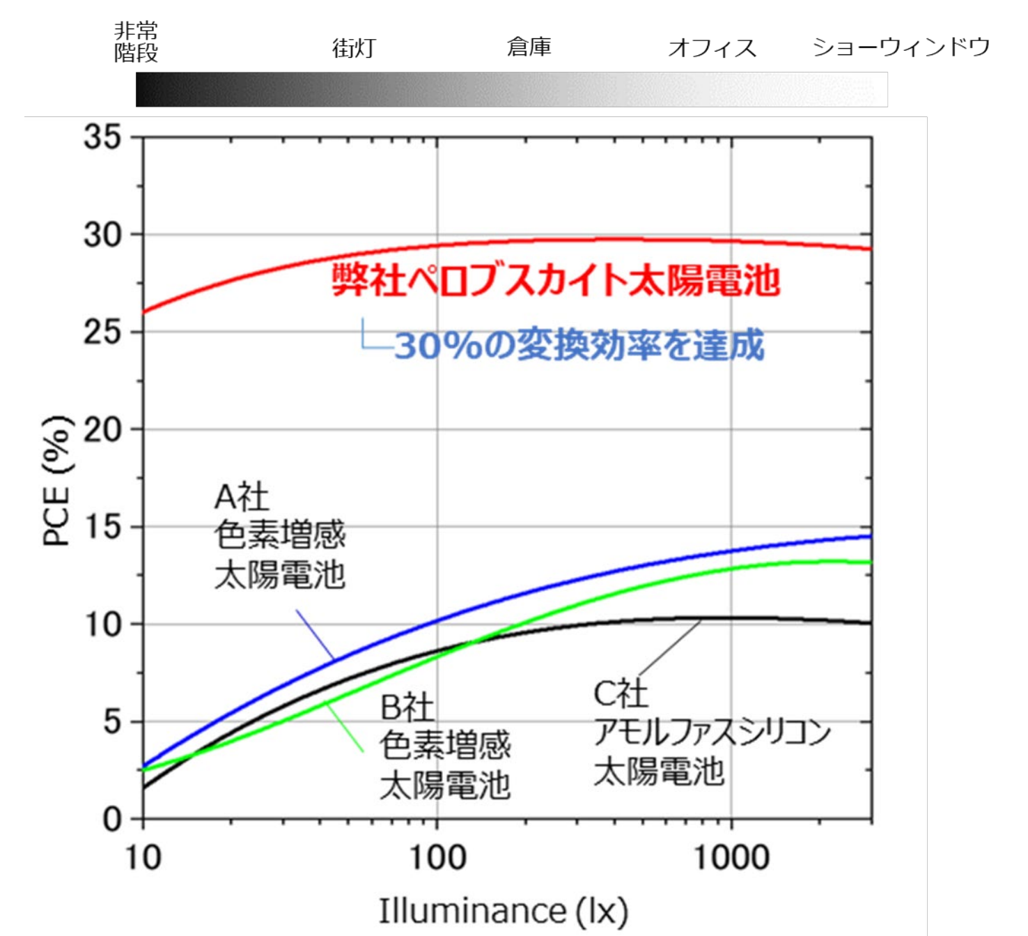
図4 照度依存特性
